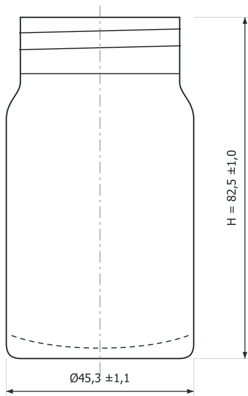
VISTA FRONTALE
