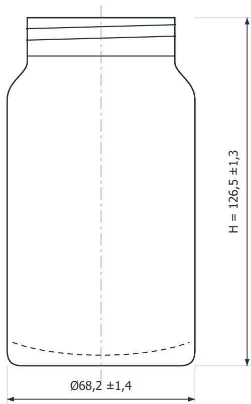
VISTA FRONTALE
