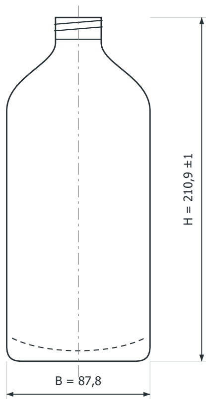
VISTA FRONTALE
