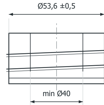
HALS — SCHEMATISCHE ANSICHT
