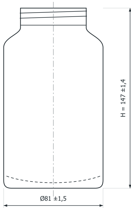
VORDERANSICHT
