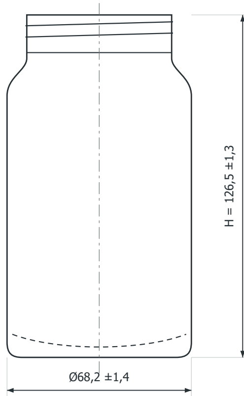
VORDERANSICHT
