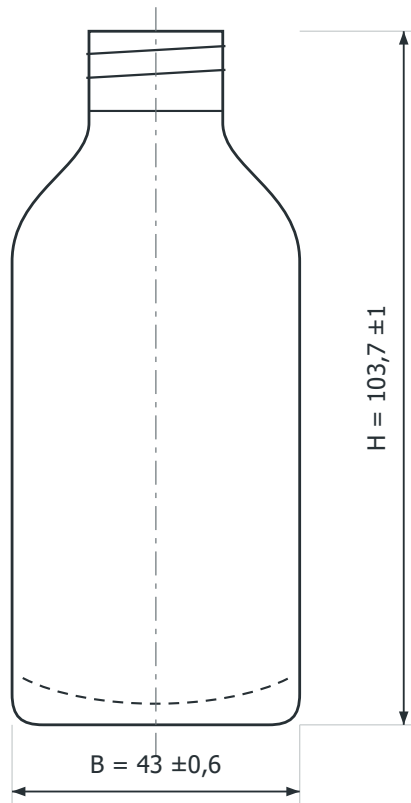
VORDERANSICHT
